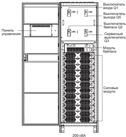
Рисунок 9 – Компоненты системного шасси ИБП серии ELECTRA OM 200 кВА
